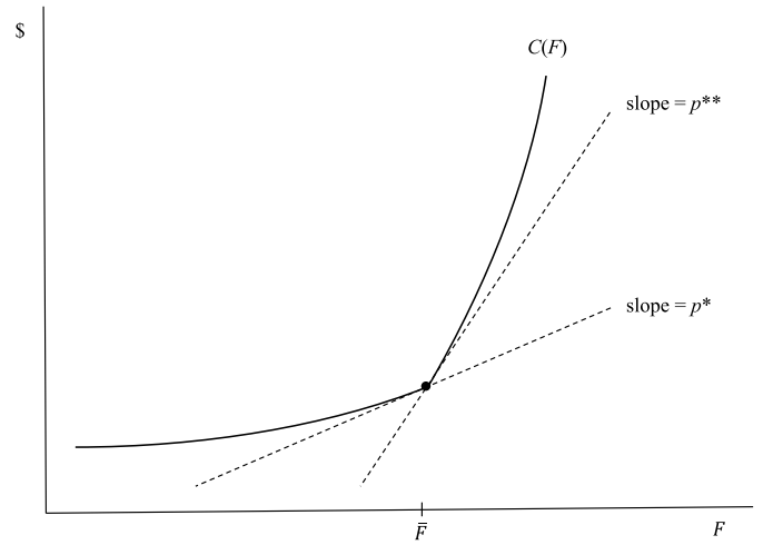
Fig. 1. Kink in C(F) .
